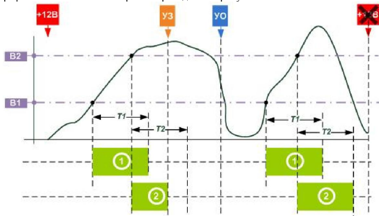
Рисунок 3 – Графическое описание алгоритма для функции 2.
