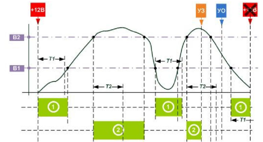
Рисунок 2 – Графическое описание алгоритма для функции 1.
