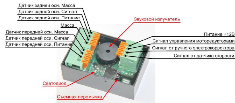
Рисунок 1 – Внешний вид блока управления автоматического корректора света фар СИЛИЧЬ-ЗЕНИТ.
