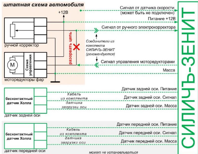
Рисунок 2 – Типовая схема подключения автоматического корректора света фар
