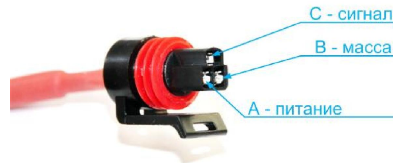
Рисунок Б.1 Вид разъема датчика загрузки спереди.
