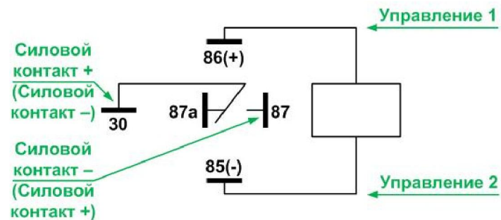
Рисунок 2 – Типовая схема подключения электронного реле «СИЛИЧЬ-ЭЛ-РЕЛЕ-П-10А».
