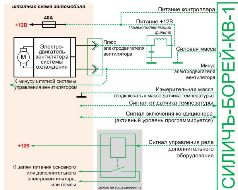
Рисунок 2 – Типовая схема подключения блока управления ЭВСО «СИЛИЧЬ-БОРЕЙ-КВ-1»
