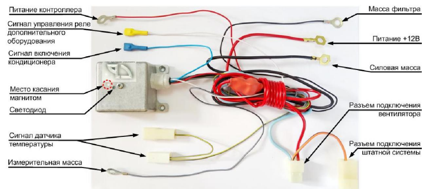
Рисунок 1 – Внешний вид блока управления ЭВСО «СИЛИЧЬ-БОРЕЙ-КВ-1»
