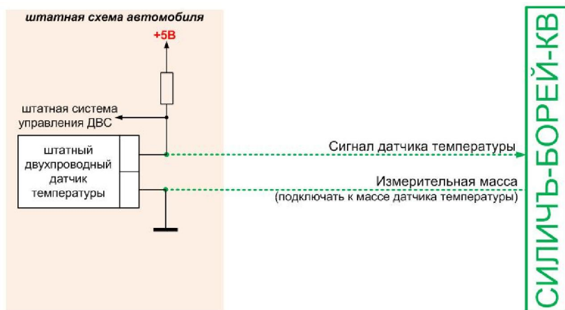
Рисунок А.1 – Схема подключения устройства к двухконтактному ДТ
