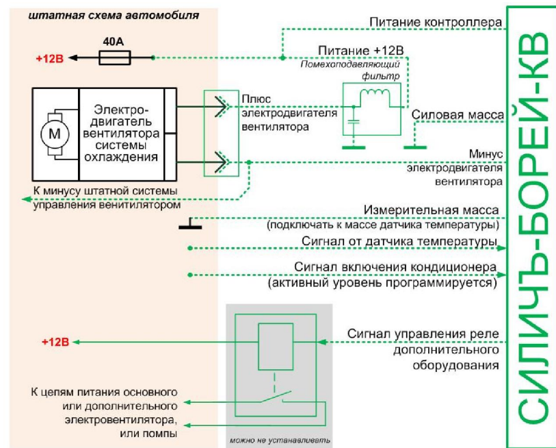
Рисунок 2 – Типовая схема подключения блока управления ЭВСО «СИЛИЧЬ-БОРЕЙ-КВ»
