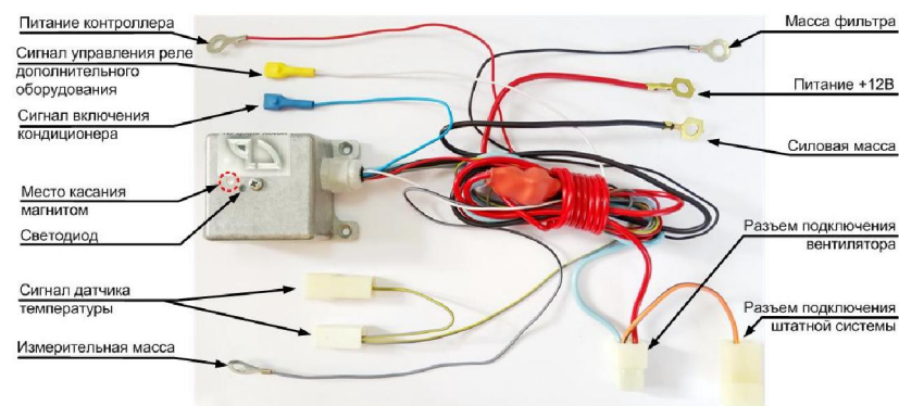
Рисунок 1 – Внешний вид блока управления ЭВСО «СИЛИЧЬ-БОРЕЙ-КВ»
