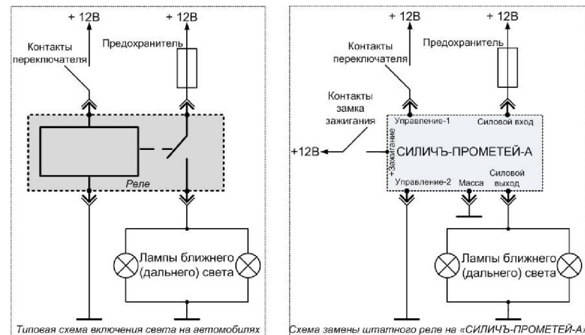
Рисунок 2 – Типовая схема подключения устройства плавного включения фар «СИЛИЧЬ-ПРОМЕТЕЙ-А» с включением реле подачей «+12В».
