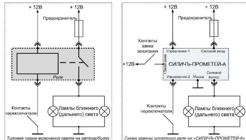
Рисунок 3 – Типовая схема подключения устройства плавного включения фар «СИЛИЧЬ-ПРОМЕТЕЙ-А» с включением реле замыканием на «массу».
