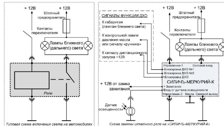
Рисунок 2 – Типовая схема подключения контроллера фар «СИЛИЧЬ-МЕРКУРИЙ-К» с включением реле подачей «+12В».
