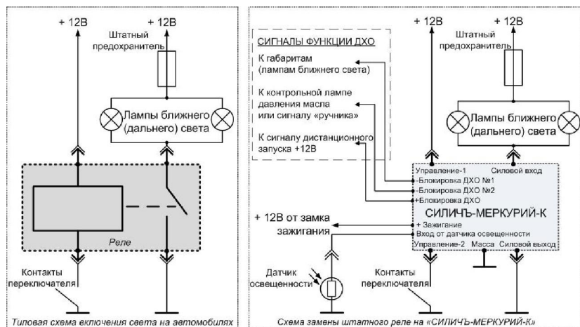
Рисунок 3 – Типовая схема подключения контроллера фар «СИЛИЧЬ-МЕРКУРИЙ-К» с включением реле замыканием на «массу».
