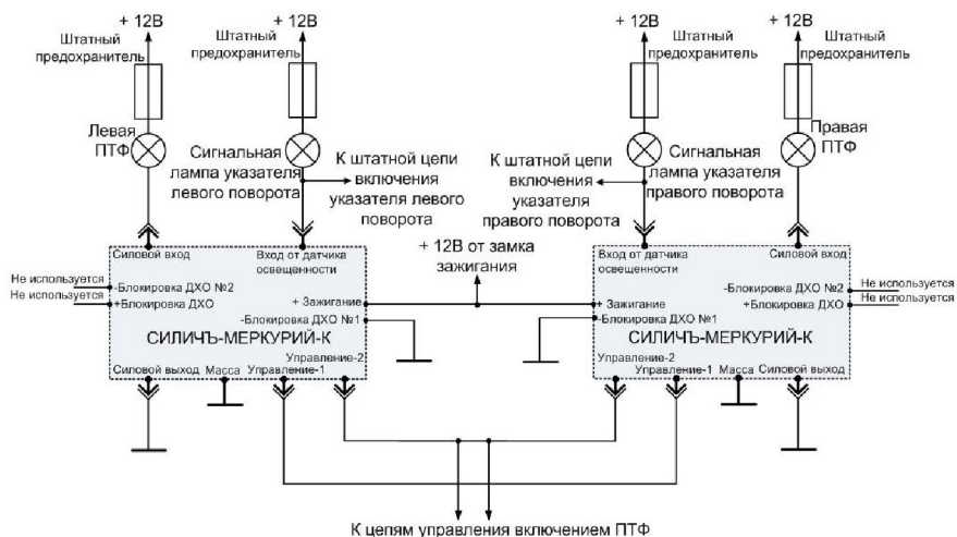
Рисунок 4 – Схема подключения двух контроллеров фар «СИЛИЧЬ-МЕРКУРИЙ-К» к ПТФ для подсветки дороги в сторону поворота.
