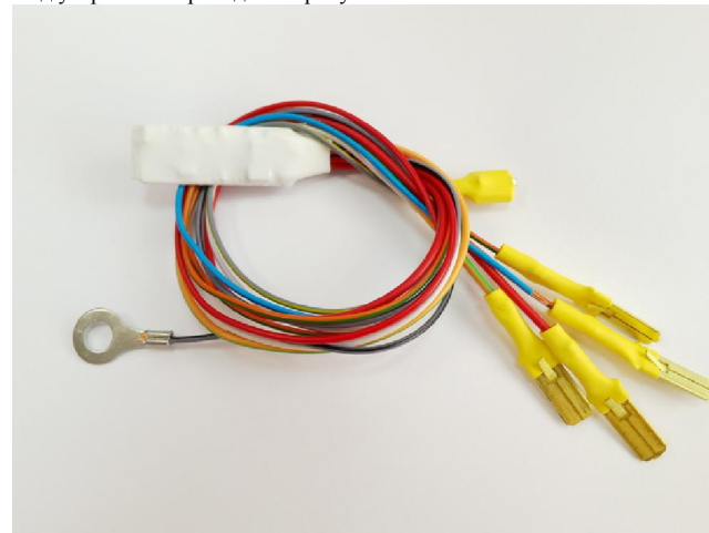
Рисунок 1 – Внешний вид контроллера фар «СИЛИЧЬ-МЕРКУРИЙ-К».
