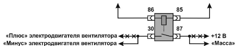
Рисунок 5 – Доработка штатной системы с коммутацией плюсового провода
