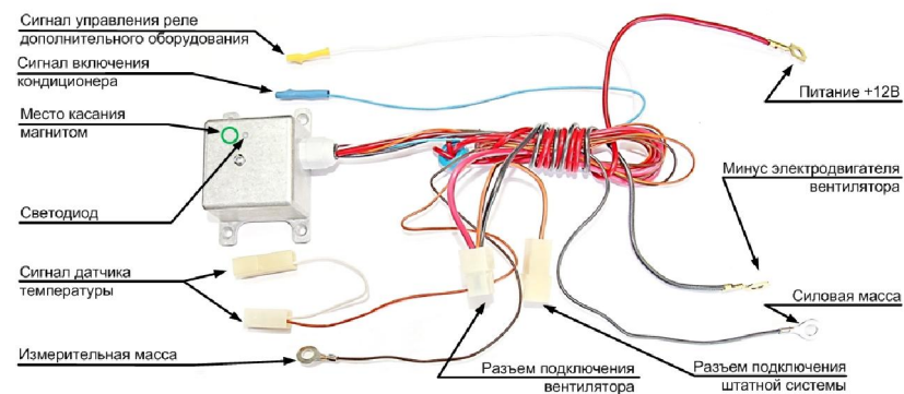
Рисунок 1 – Внешний вид блока управления ЭВСО «СИЛИЧЬ-БОРЕЙ-АВ»
